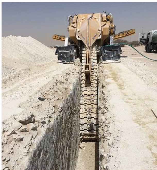
ترنچر- Trencher
