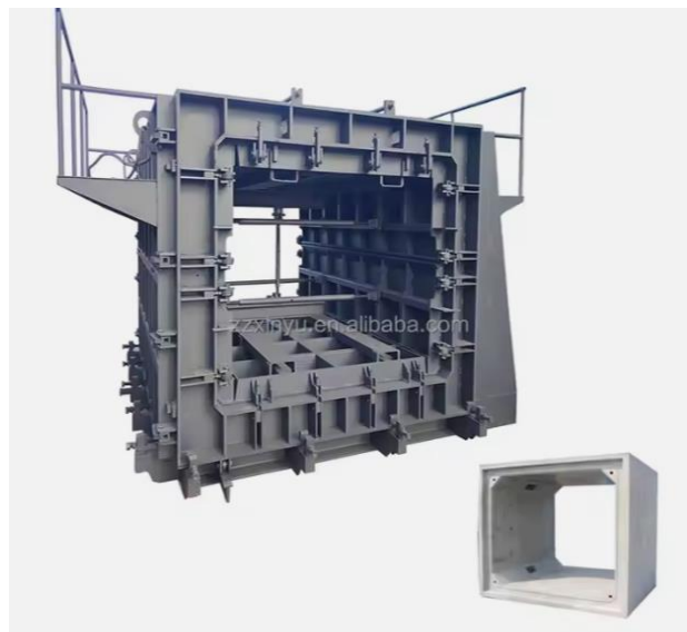
قالب تونلی
