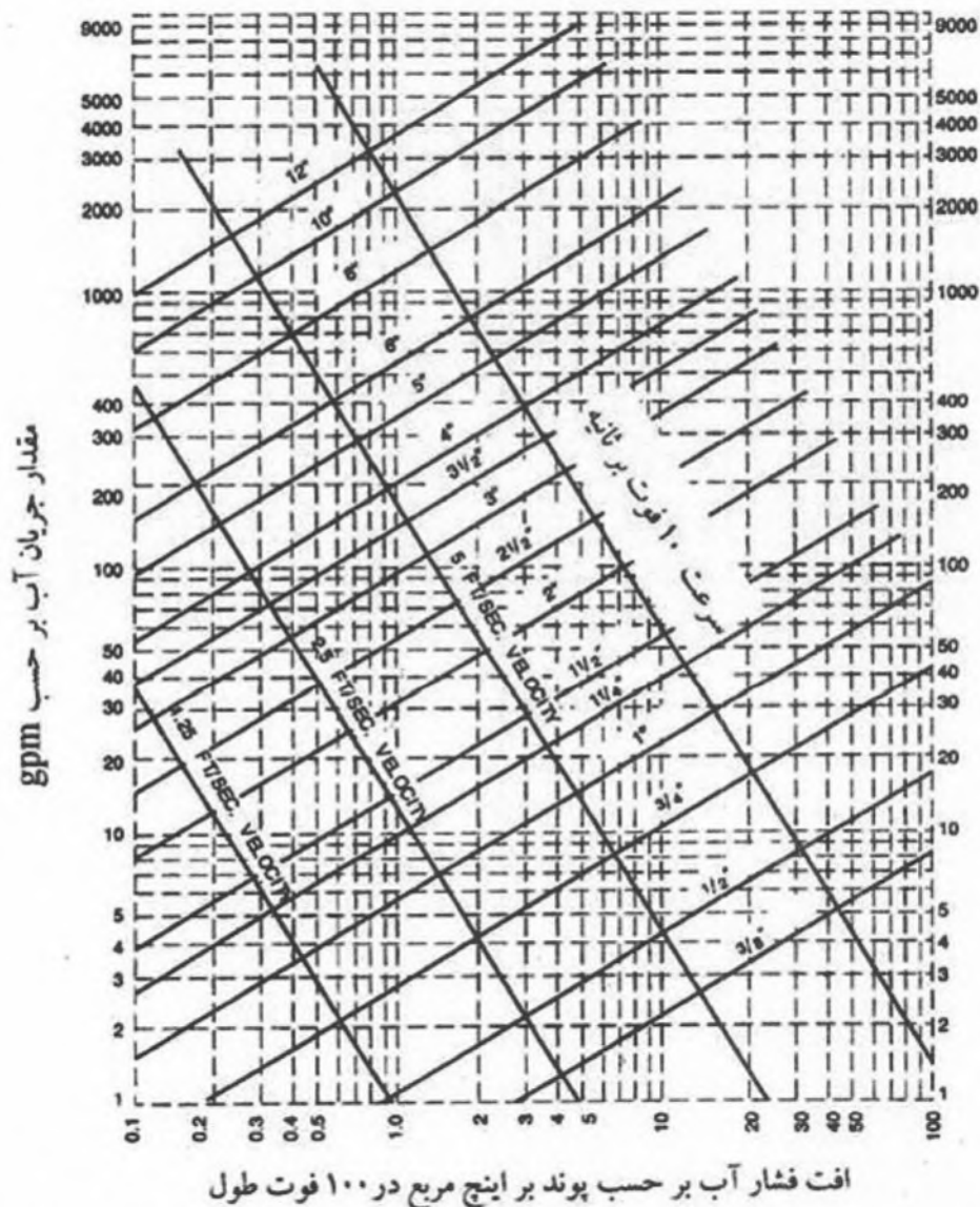
شکل پ ۷-۵-۱ (IP) منحنی اندازه‌گذاری لوله‌های مسی نوع M از استاندارد ASTM B 88
