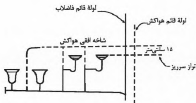
شکل ۵-۱۶-۲-۵ پ"پ (۲)- اتصال هواکش به شاخه افقی لوله فاضلاب
