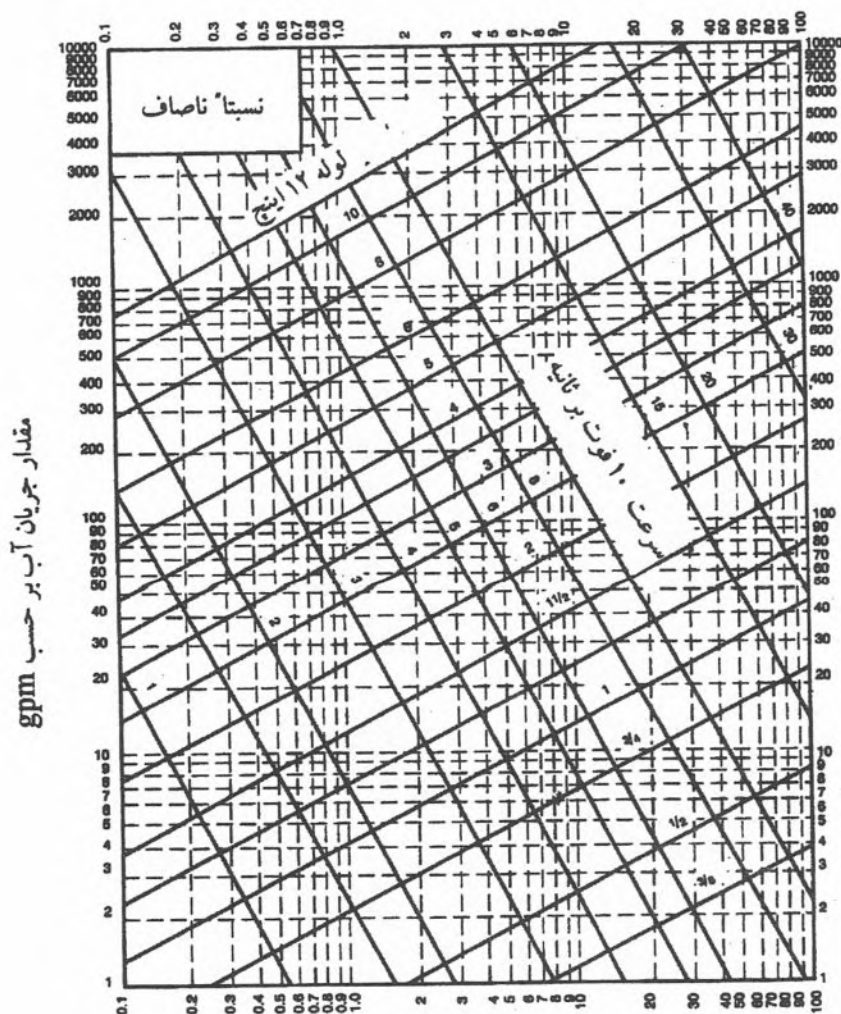
افت فشار آب بر حسب فوت در اینچ مربع در ۱۰۰ فوت طول
