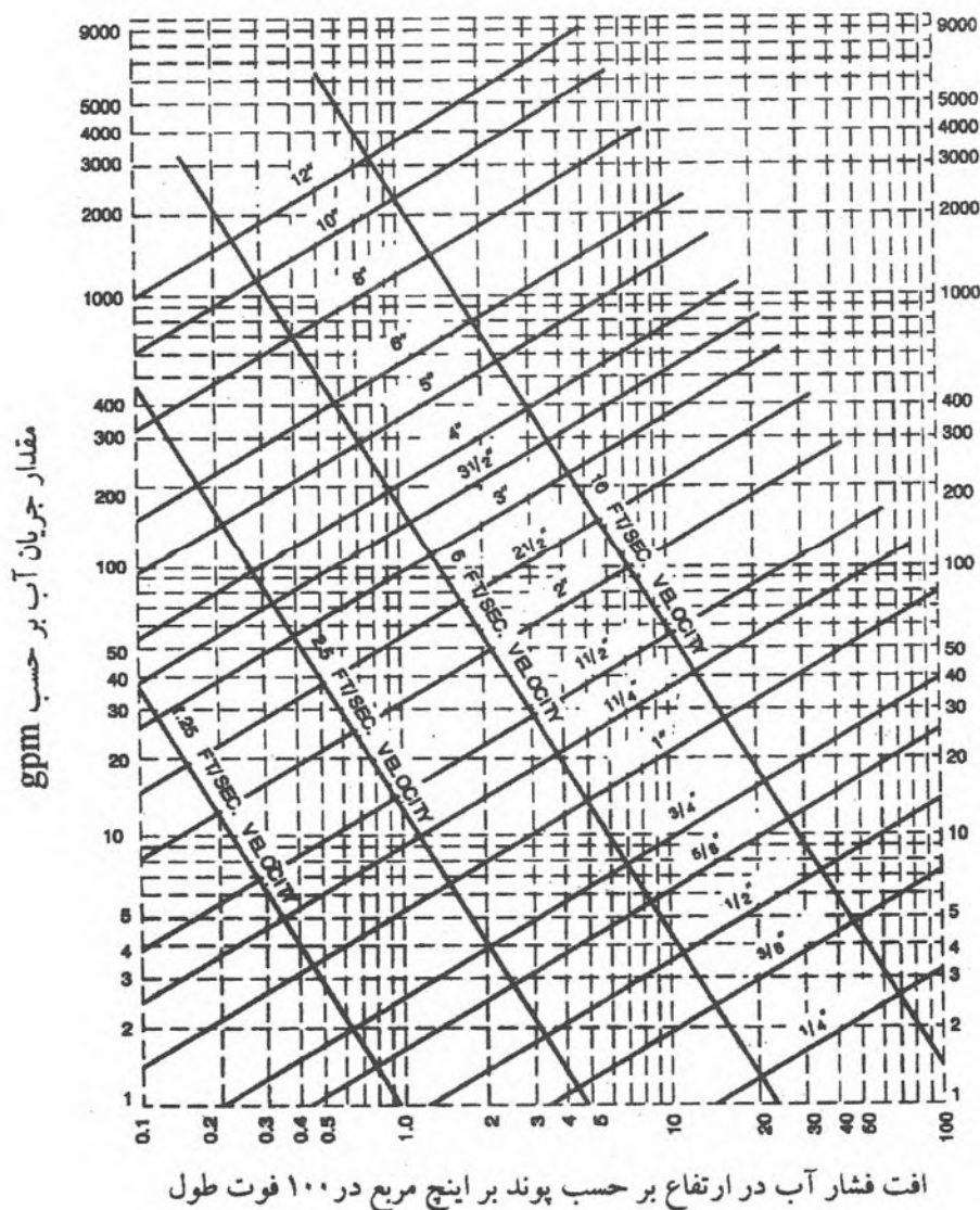
شکل پ ۱-۵-۶ (IP) منحنی اندازه‌گذاری لوله‌های مسی نوع L از استاندارد ASTM B 88
