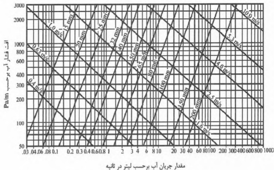
شکل پ ۱-۵-۸- (SI) منحنی اندازه‌گذاری لوله‌های پلاستیکی
