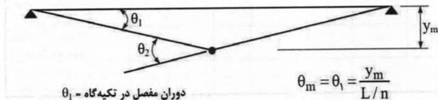
شکل ۵-۵-۲۱ - دوران مفصل خمیری
