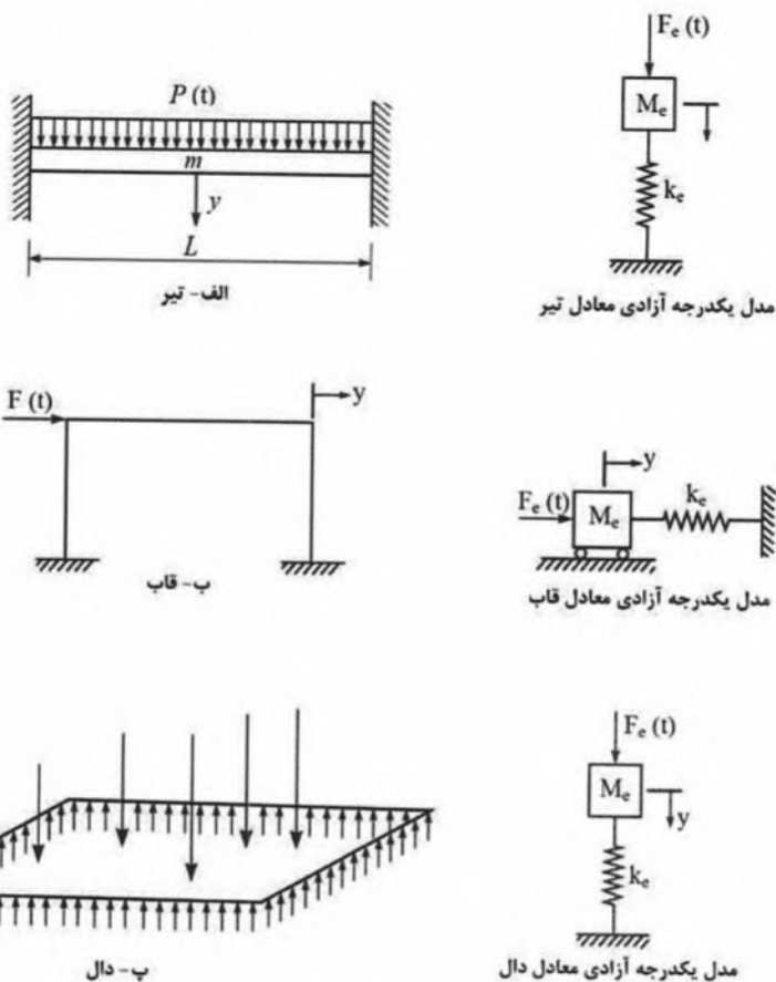
شکل ۲۱-۵-۱- معادل سازی سازه ها با مدل یک درجه آزادی
