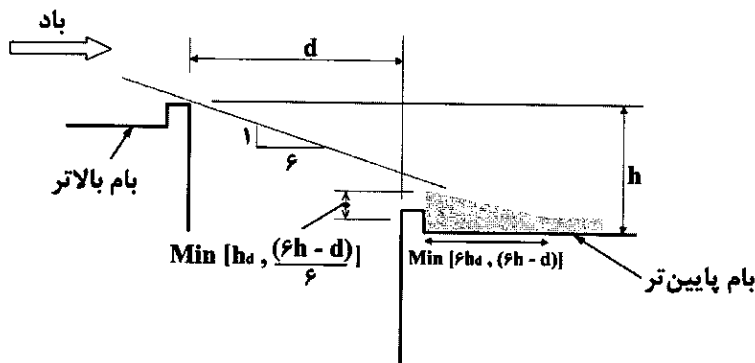
شکل ۶-۷-۹-۲ بار انباشتگی برف پشت به باد روی بام پایین‌تر ساختمان مجاور
