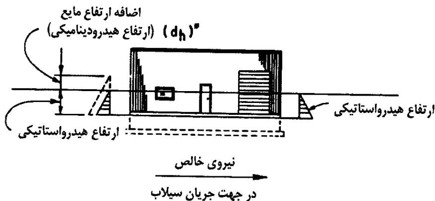
شکل ۶-۶-۲ نیروهای هیدرواستاتیکی و هیدرواستاتیکی در جهت جریان سیلاب
